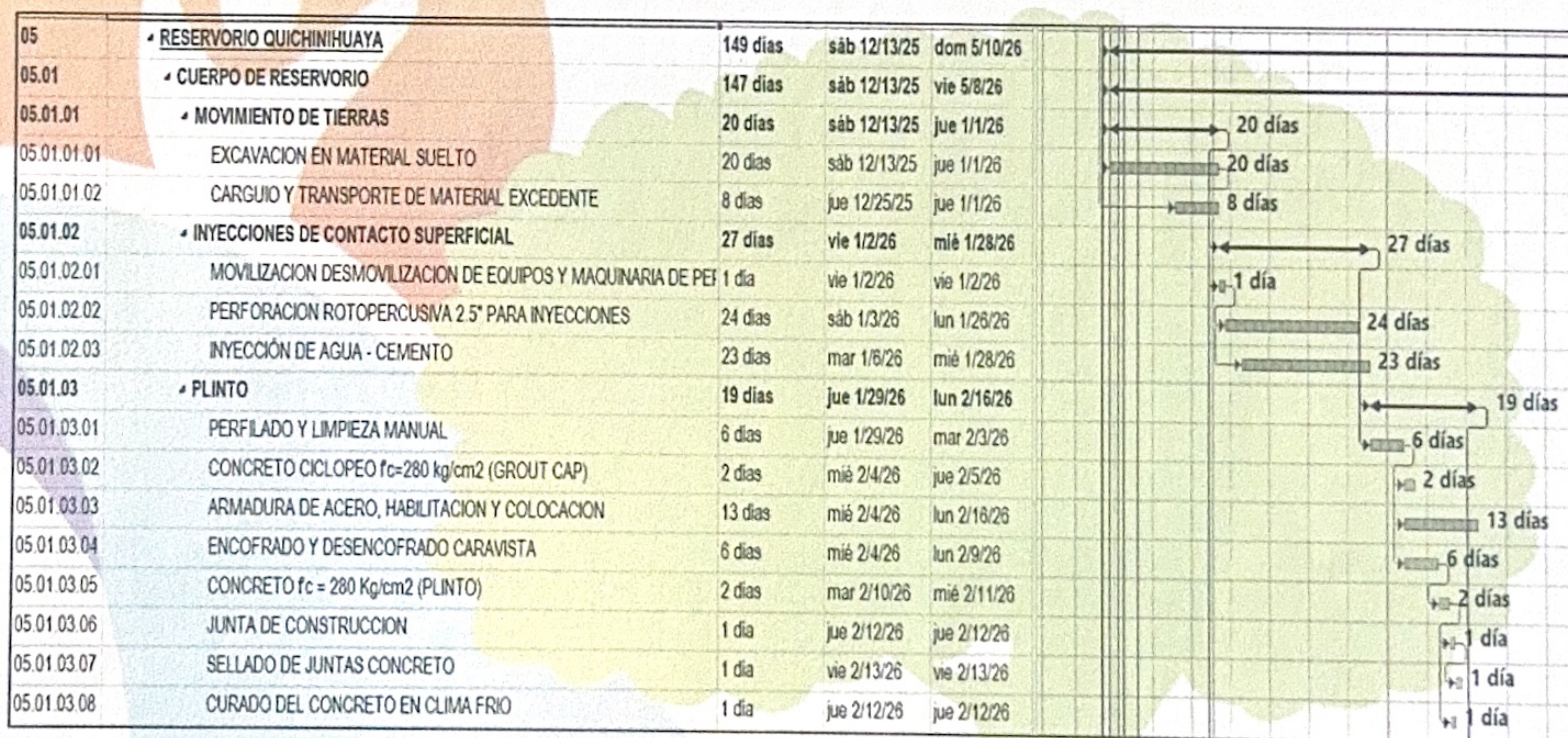
Extraído del cronograma GANTT actualizado de obra
